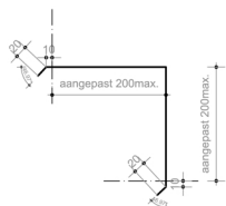
HOEK PROFIEL AANGEPAST /86
