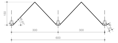
PROFIEL 86x2 /125
