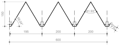
PROFIEL 62hoek x3 /62
