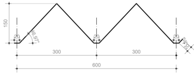
PROFIEL 86x2 /86
