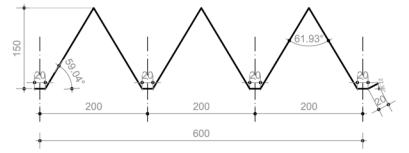
PROFIEL 62x3 /125
