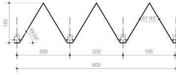
PROFIEL 62hoek x3 /0
