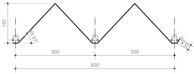
PROFIEL 86x2 /62
