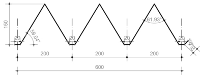
PROFIEL 62x3 /86
