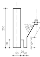
RAND PROFIEL
