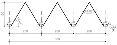
PROFIEL 62x3 /62
