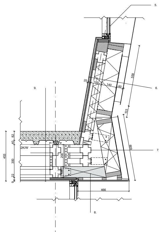
Detail V2
