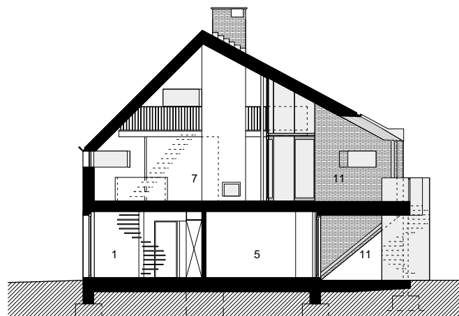
snede AA
