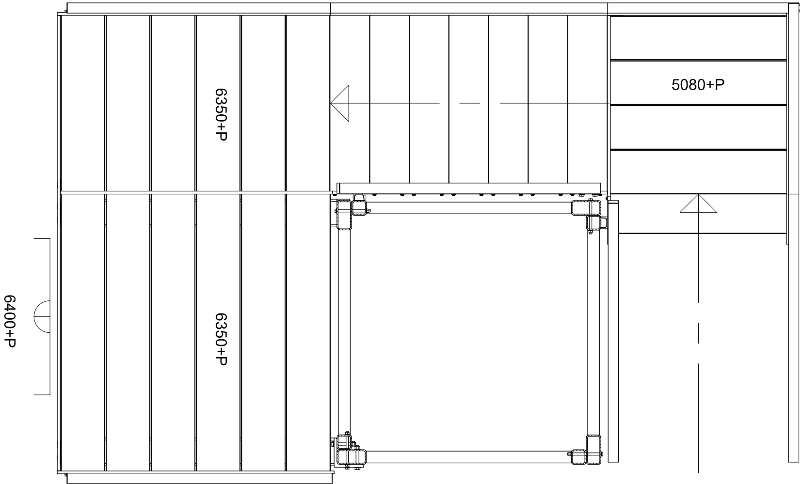
bovenaanzicht 6350+ (+1500/-1500)
