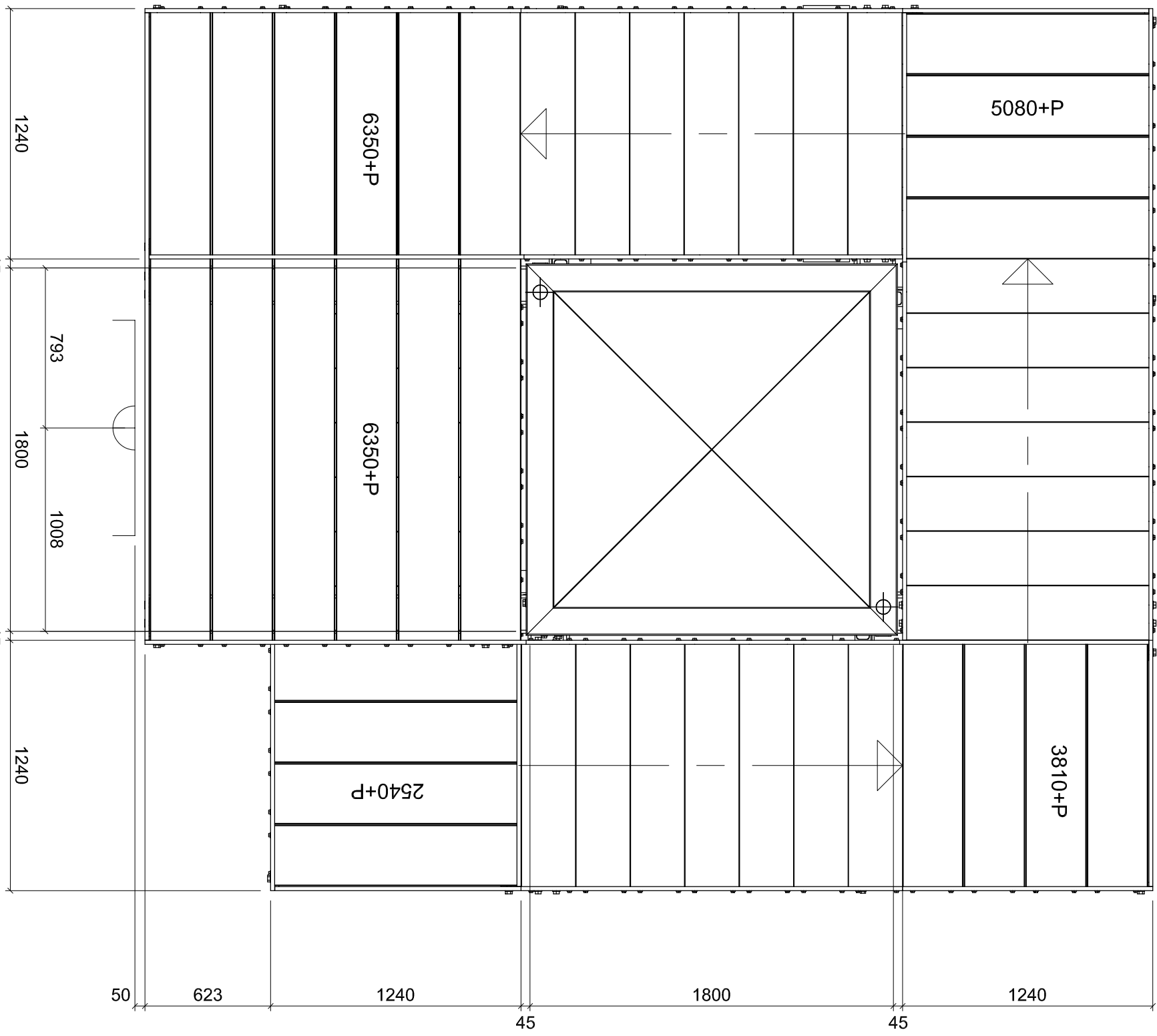
bovenaanzicht totaal
