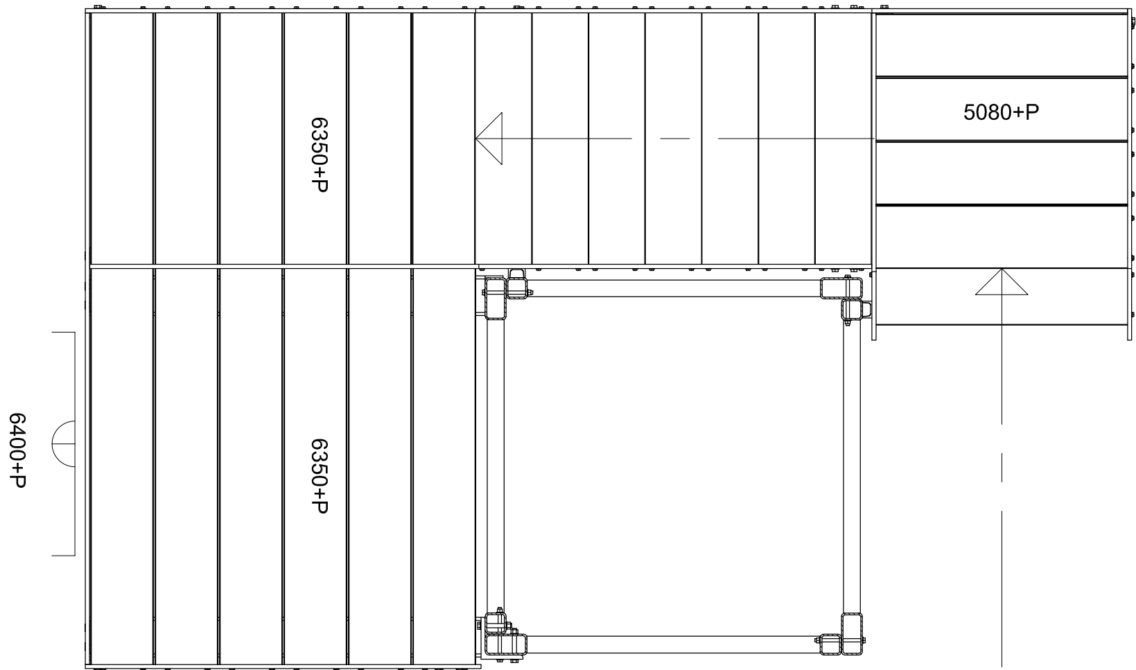
bovenaanzicht 6350+ (+500/-1500)
