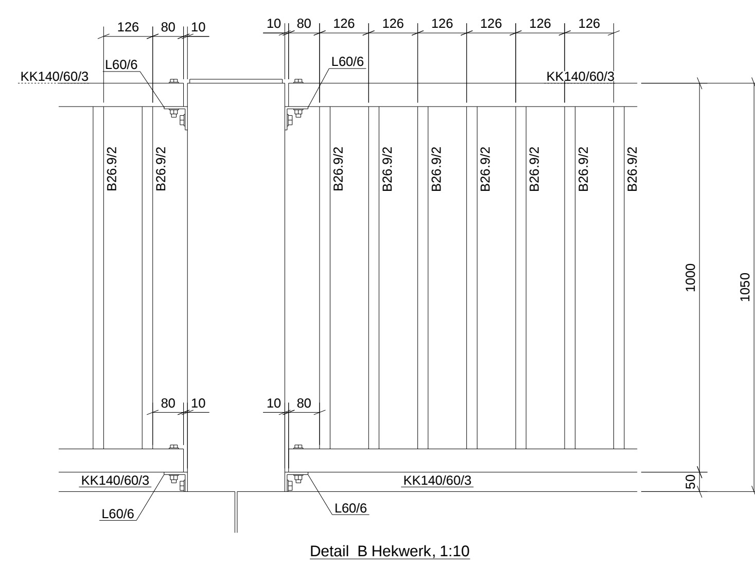
Detail B Hekwerk 1:10
