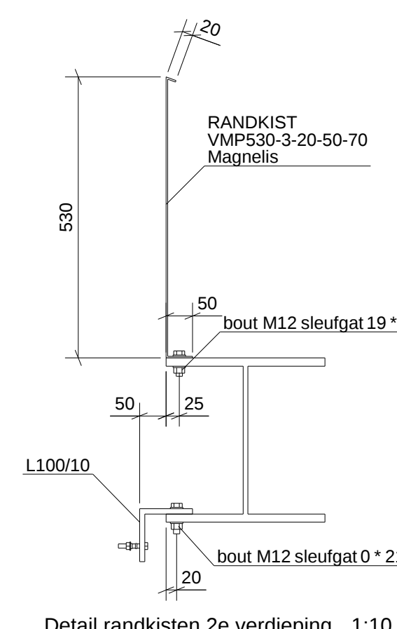
Detail randomist 2e verdieping 1:10
