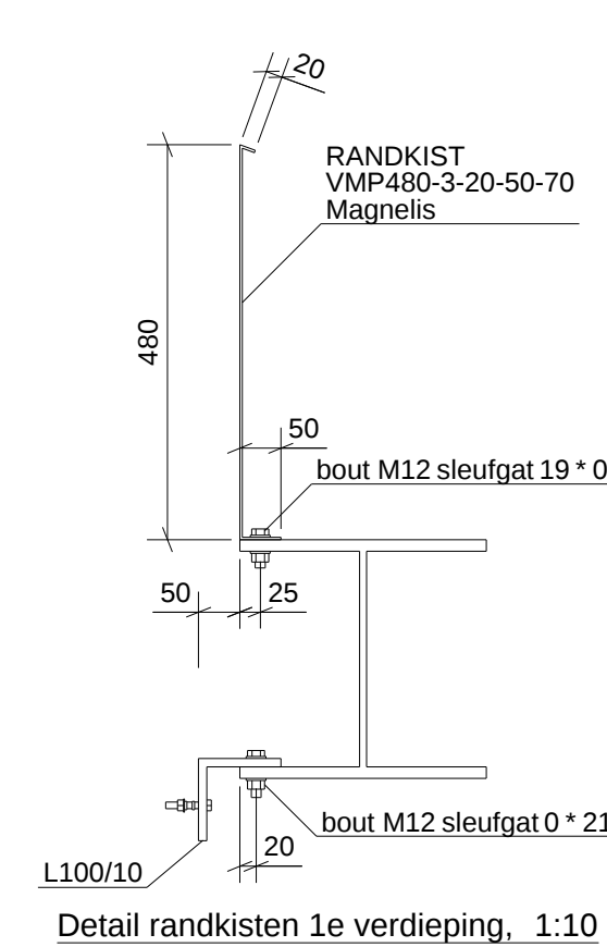
Detail randomist 1e verdieping 1:10
