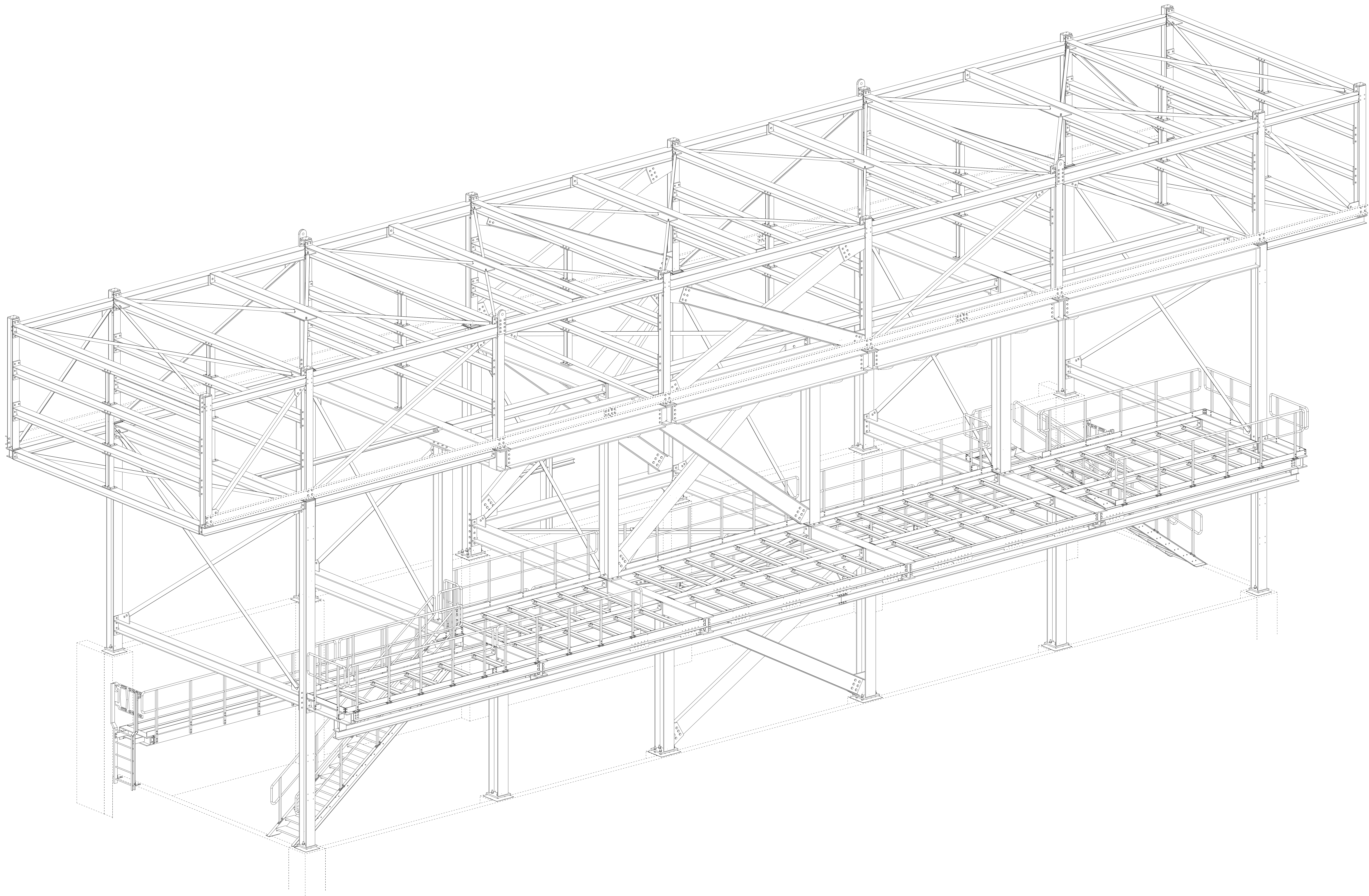
3D ZICHT SCHAAL 1:30
