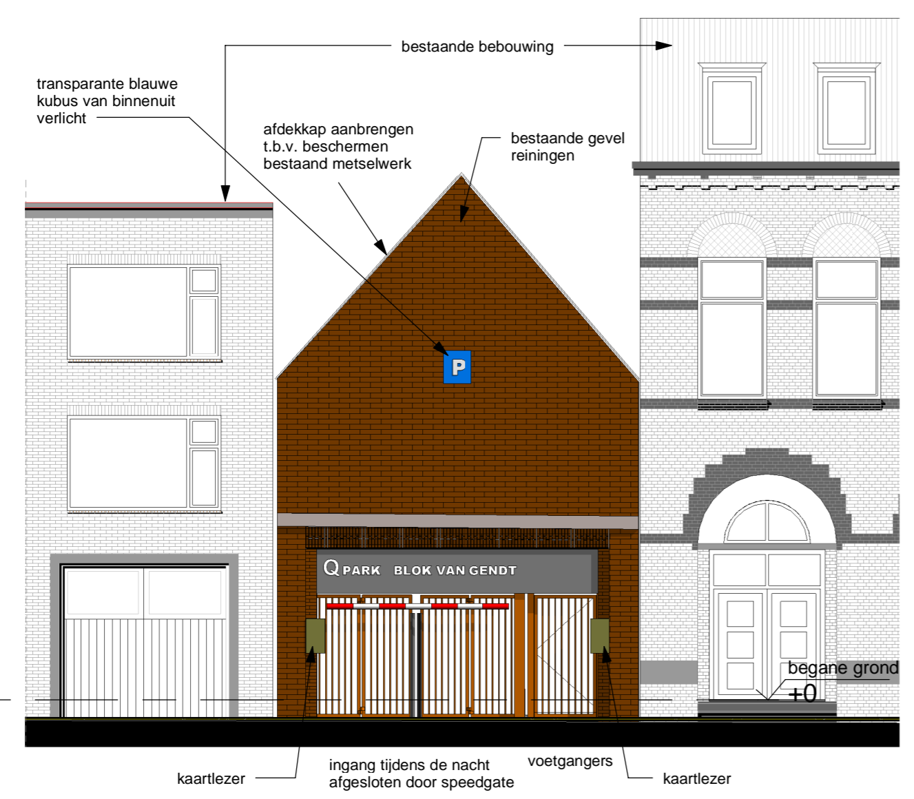
gevel Valuastraat
