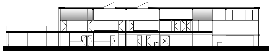
Doorsnede D-D
