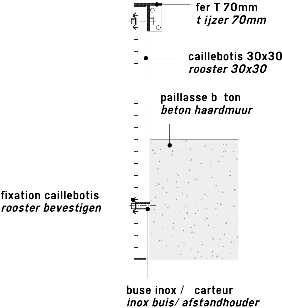
D tail fixation garde-corps lat ral escalier ext rieur en coupe Bevestigen lateraal vangrail buiten trap in snede 1:5
