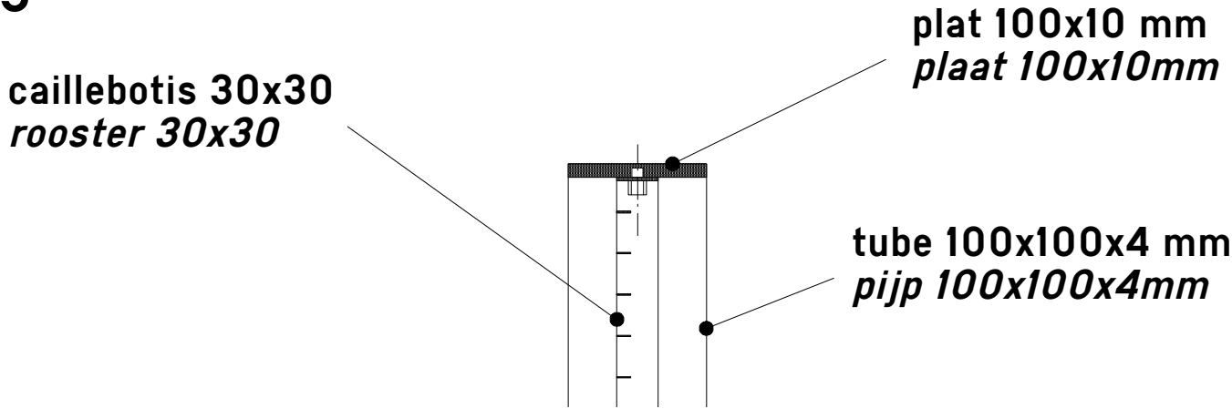
D tail haut du garde-corps central escalier ext rieur en coupe Hoog van de centraal vangrail buiten trap in snede 1:5
