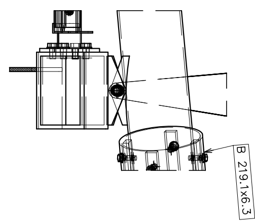
Koppeling spriet aan bordesrand
