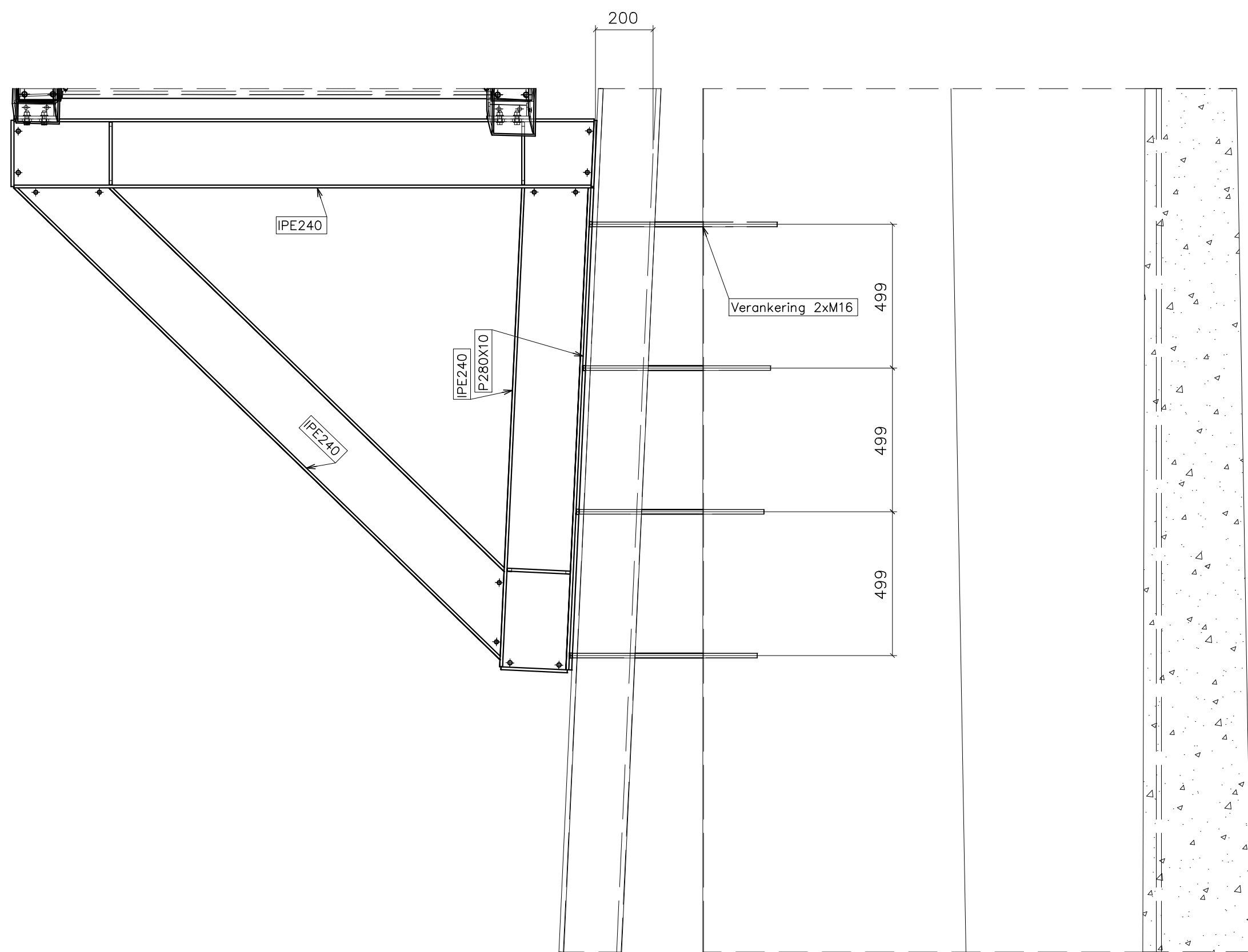
Aanzicht loopbordes support
