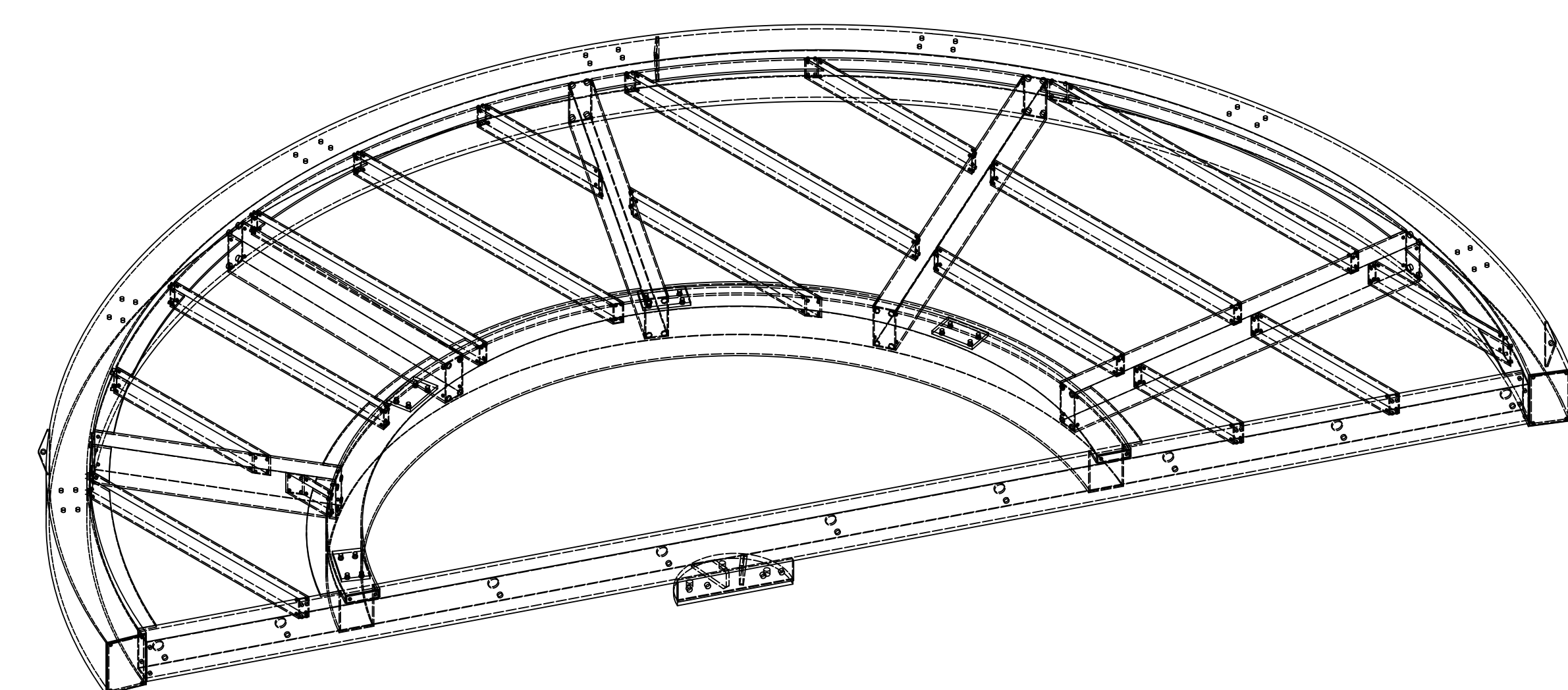
Isometrie
