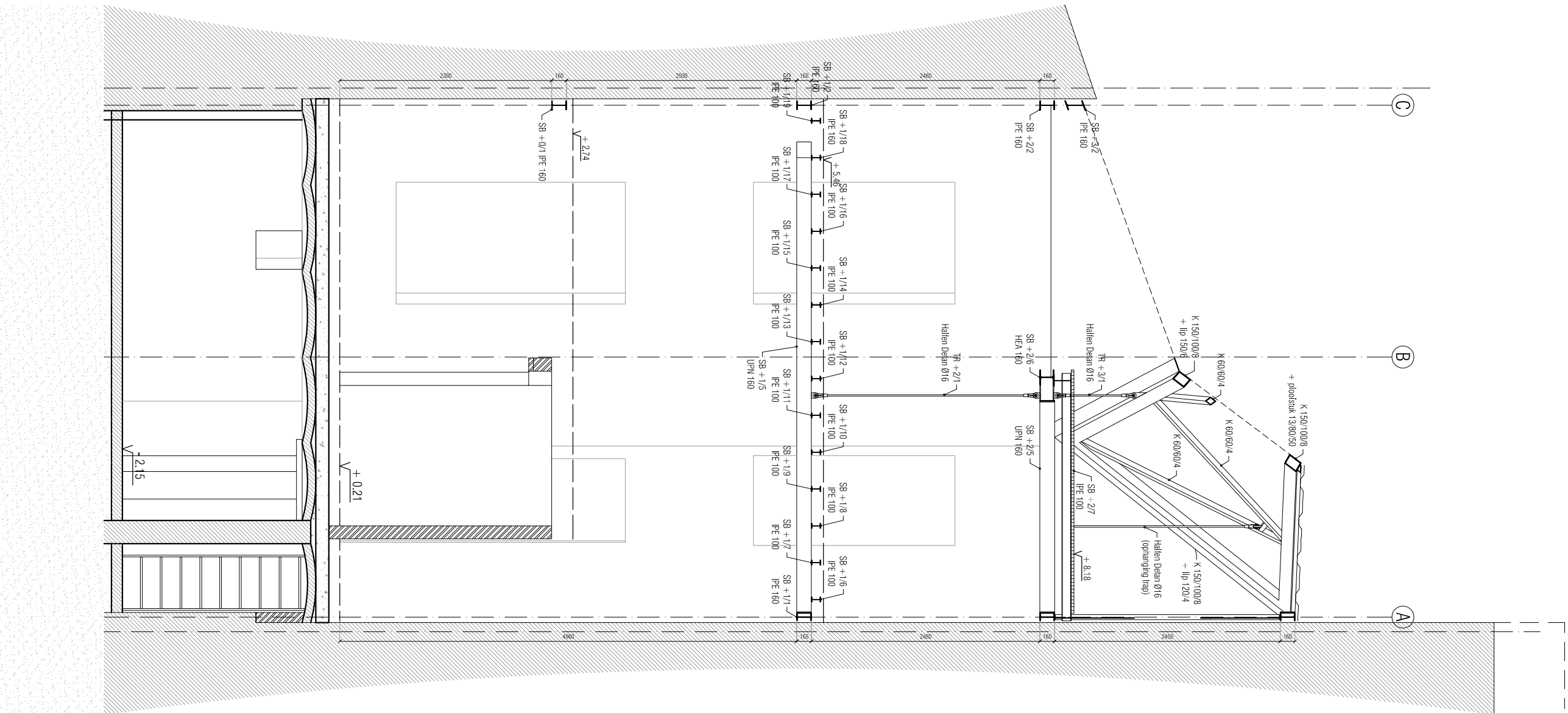
Aanzicht AS 2
