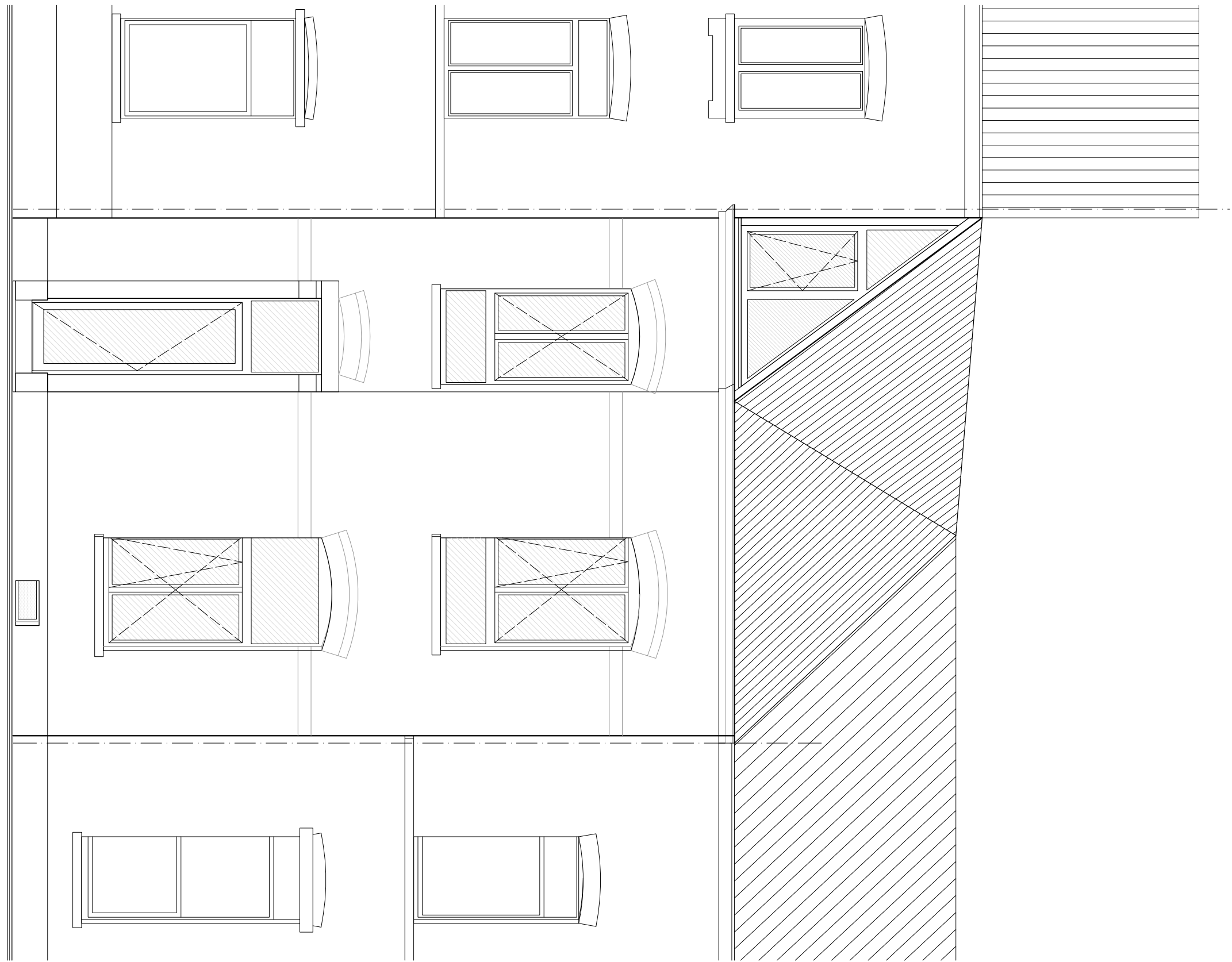
VOORGEVEL
