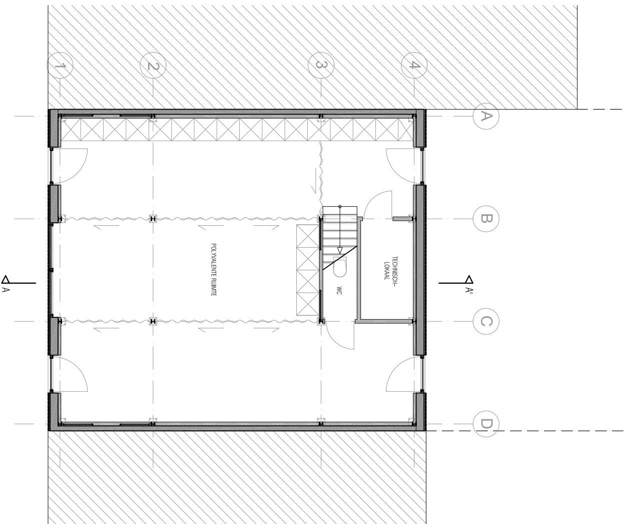
PLAN GELUKVLOERS
