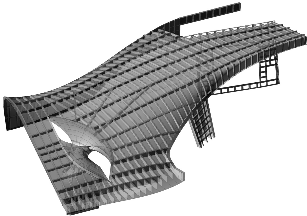
Dakconstructie bovenzijde
