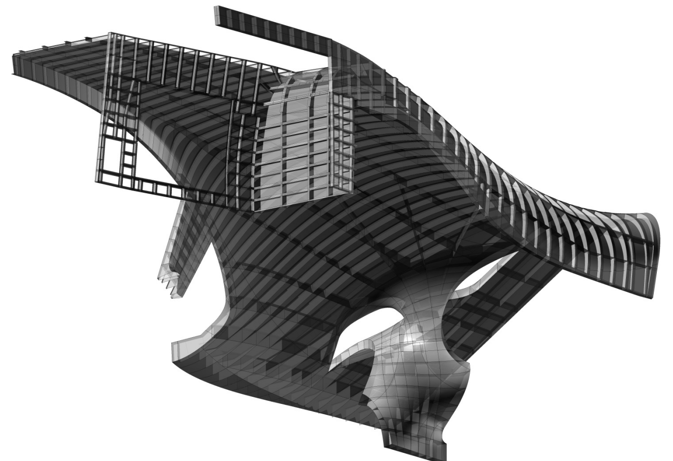
Dakconstructie onderzijde
