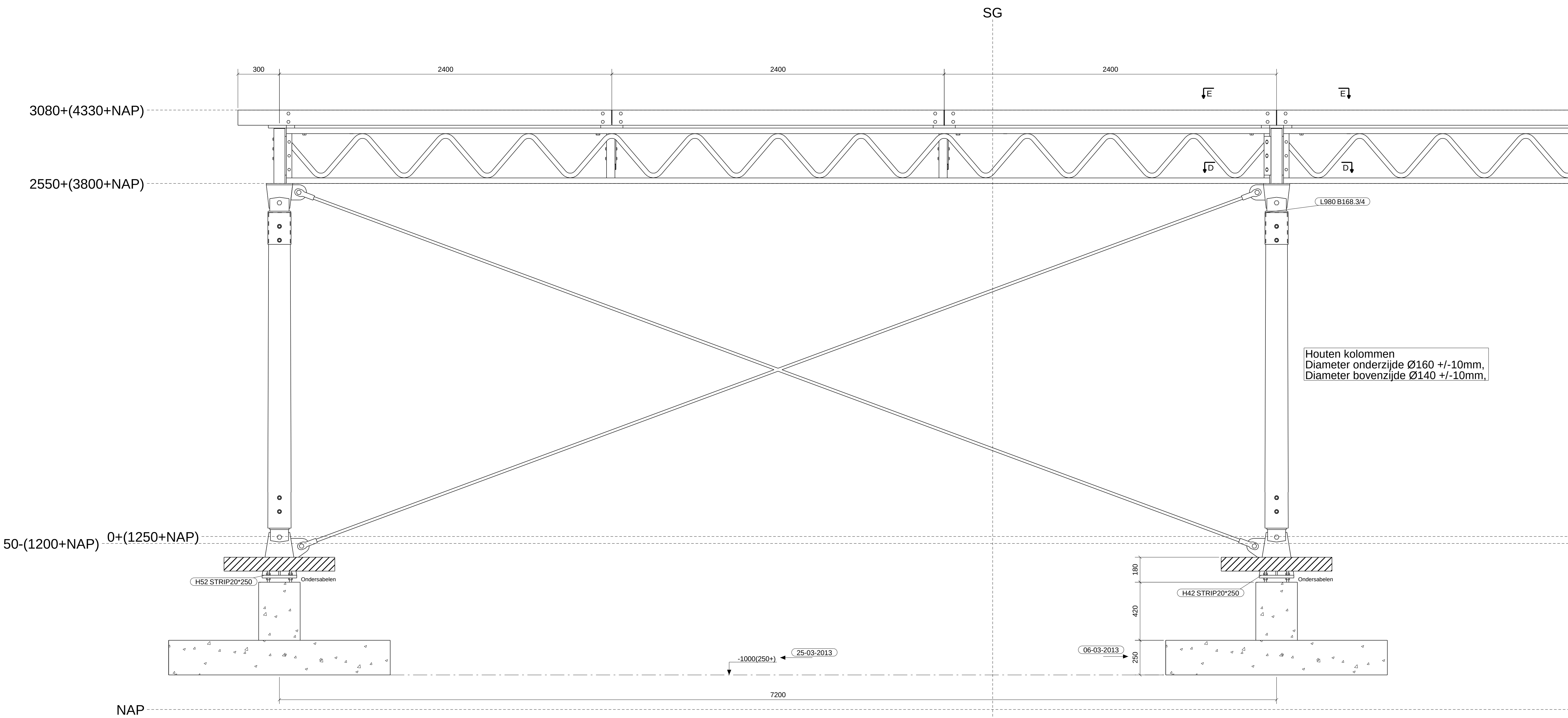
LANGSDOORSNEDE PB2 EN PB3
