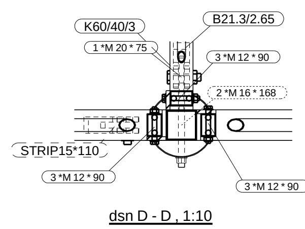
dsn D - D, 1:10
