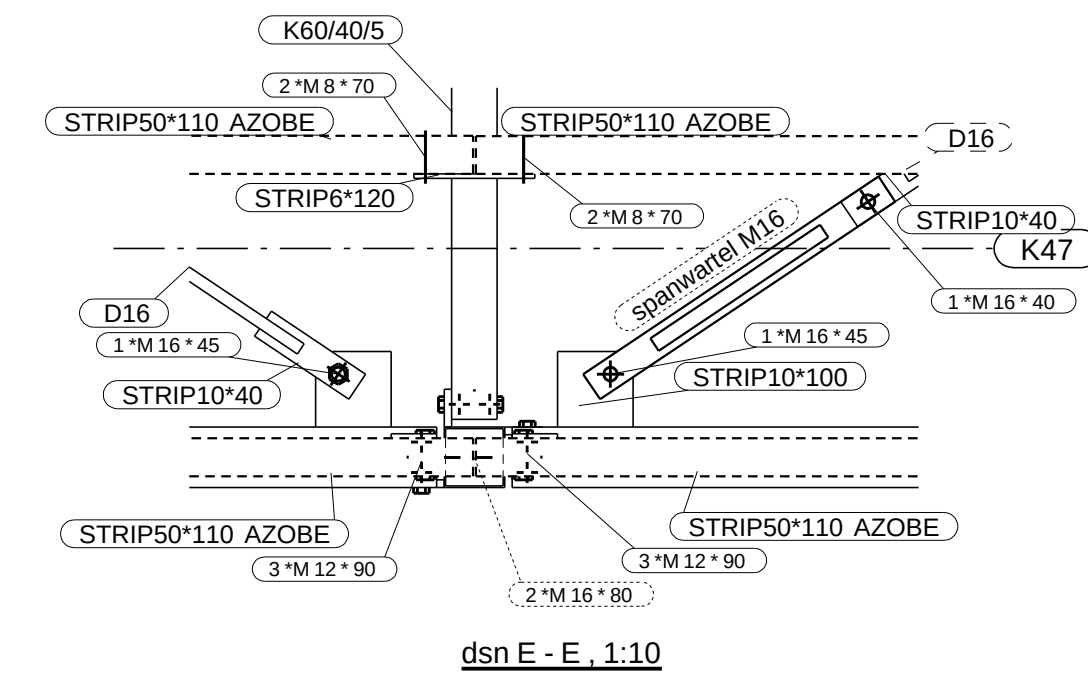
dsn E - E, 1:10
