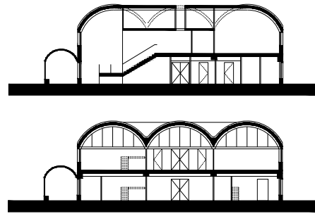
Doorsnedes
