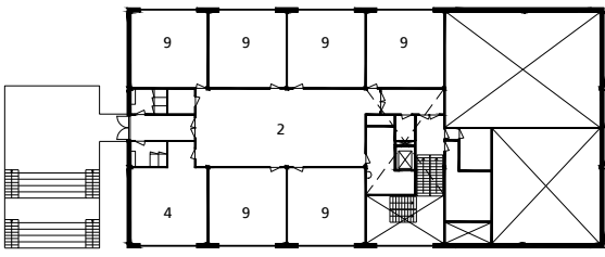
1e verdieping
