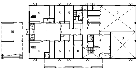
Begane grond
