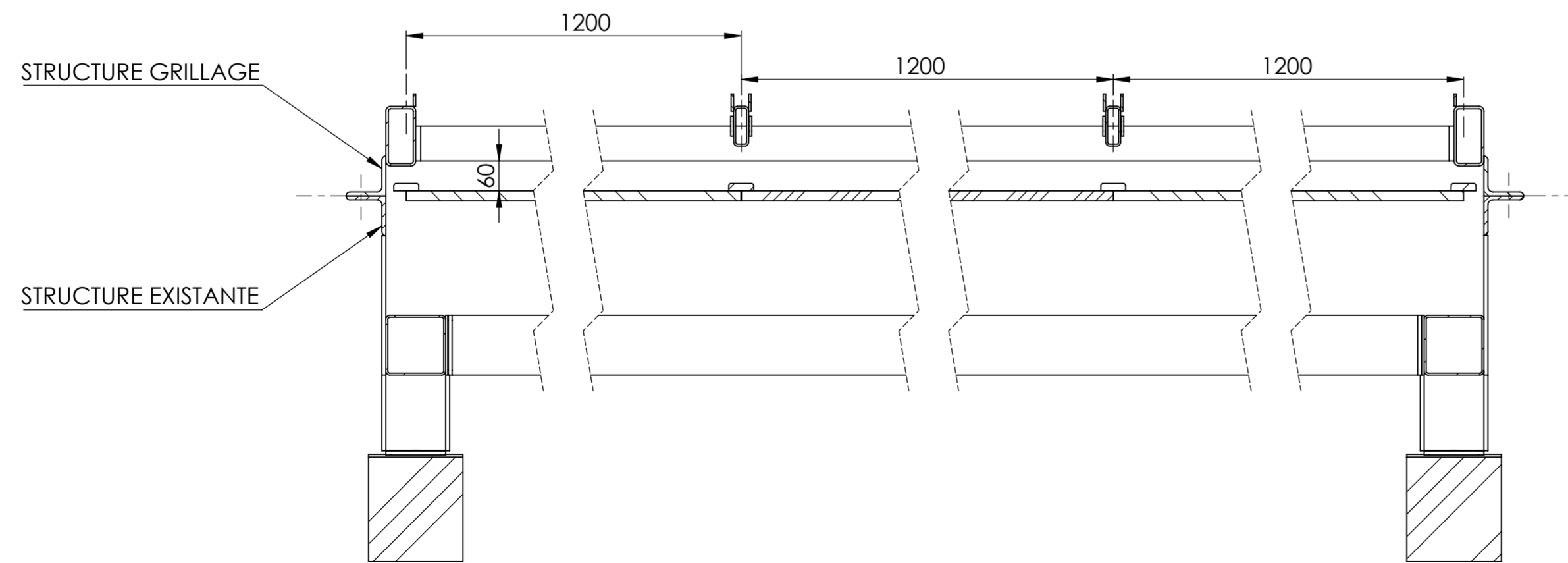
COUPE A-A ECHELLE 1 : 10
