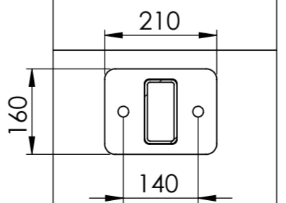
COUPE F-F DETAIL PLATS FIXATION
